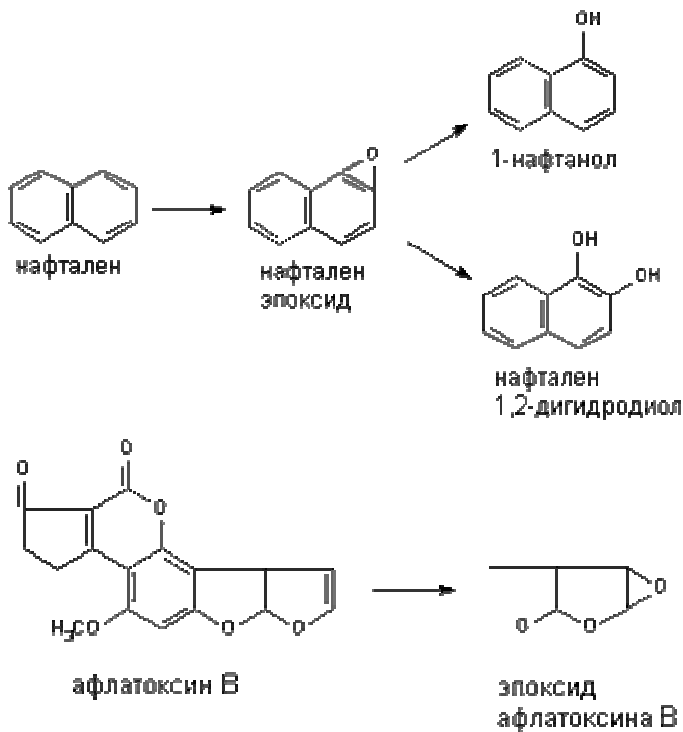
Рис. 41. Эпексидирование нафтадена и афлатоксина В, катализируемое цитохромом Р-450
