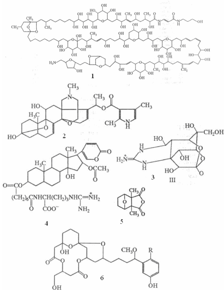
Рис. 31. Структура зоотоксинов небелковой природы: 1 — палитоксин; 2 — батрахотоксин; 3 — тетродотоксин; 4 — буфотоксин; 5 — кантаридин; 6 — аплизиятоксин ( R=Br )
